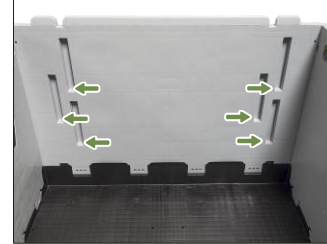
7. Arka panelin iç tarafında bulunan ara gözlerin muylularını için yuvalar.
